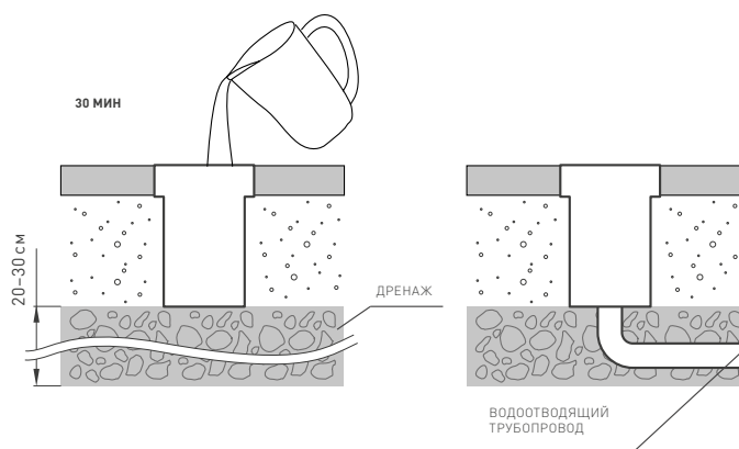
Рис. 2. Установка светильника в грунт
